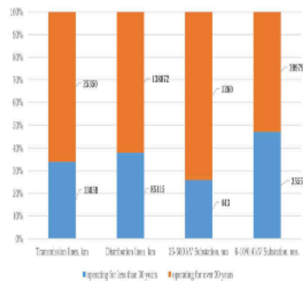
[그림2] 우즈베키스탄 송전망 현황
